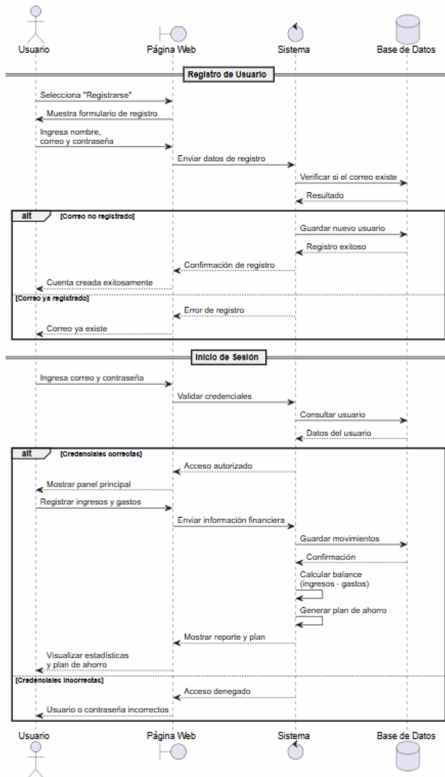
Diagrama de Secuencia - Registro e Inicio de Sesión
