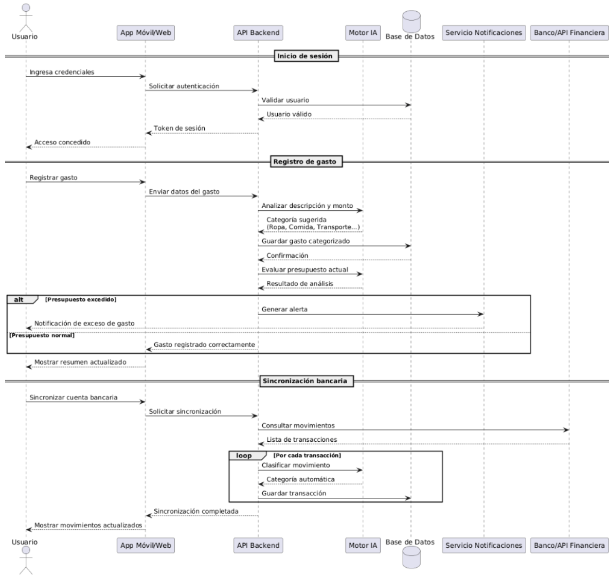
Diagrama de Secuencia - Registro Inteligente de Gastos
