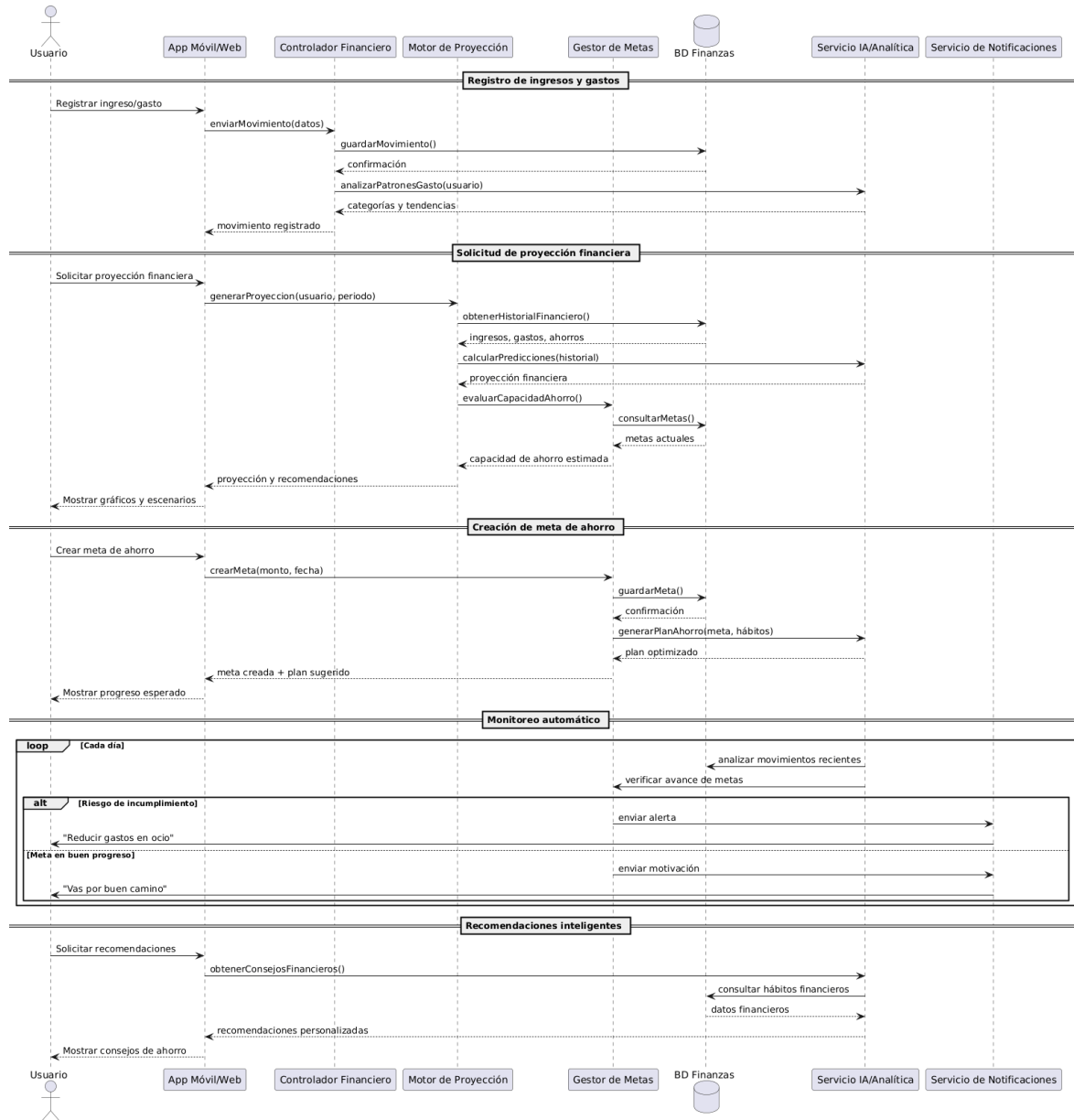
Sistema Inteligente de Control de Gastos Diagrama de Secuencia - Proyección Financiera y Metas de Ahorro
