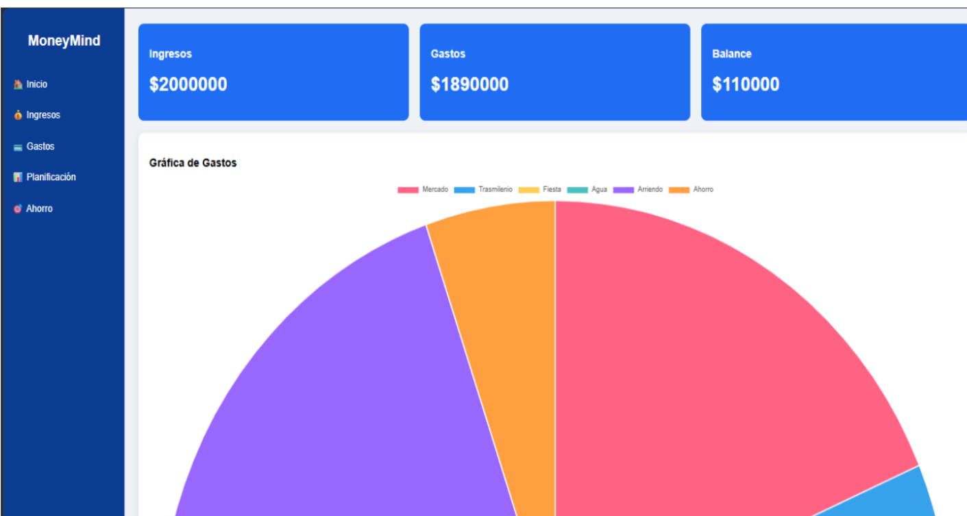
Imagen 5.-Moneymind Interfaz
